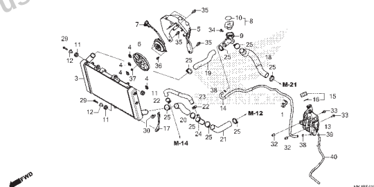
C-41 Radiador
