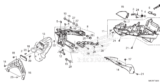
C-37 Bateria
