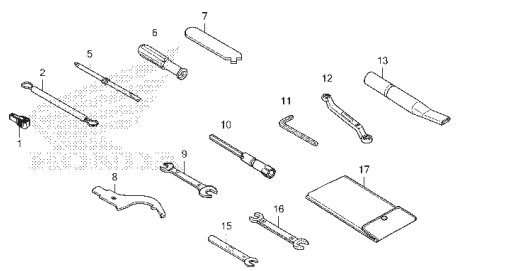
C-48 Ferramentas
