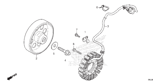
M-11 Gerador
