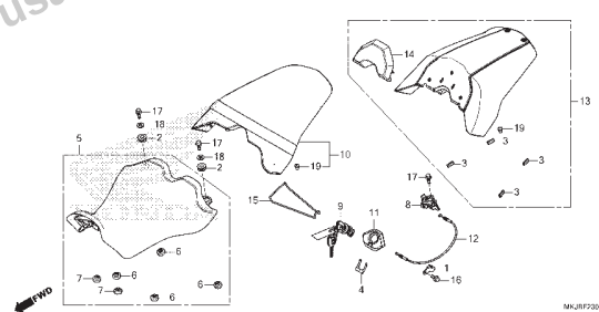
C-23 Assento
