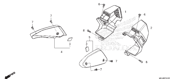
C-26 Câister
